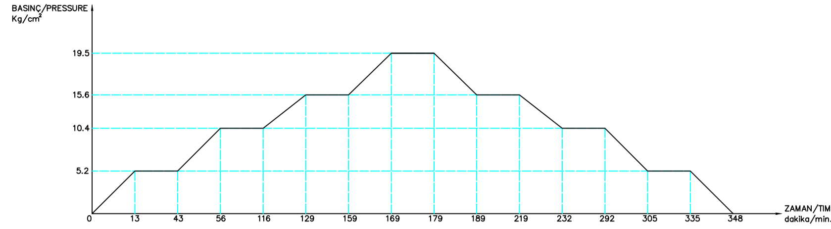
BRANSMAN BÖLÜMÜ TESTİ BASINÇ/ZAMAN DIAGRAMI WYE BRANCH SECTION TESTING PRESSURE/TIME DIAGRAM
