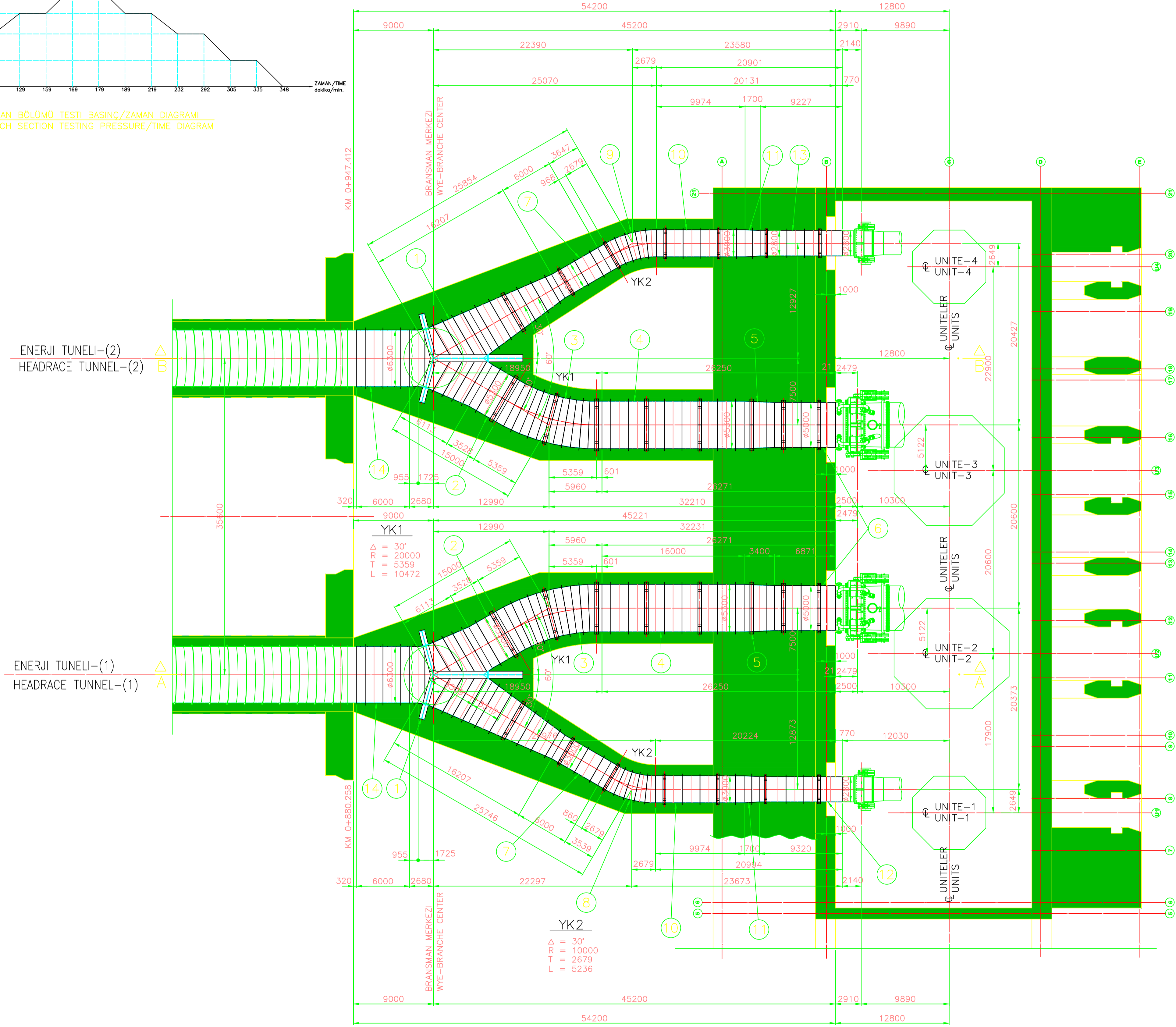
BRANSMAN BOLGESI PLANI WYE-BRANCHE PLAN ÖLÇEK=SCALE: 1/250
